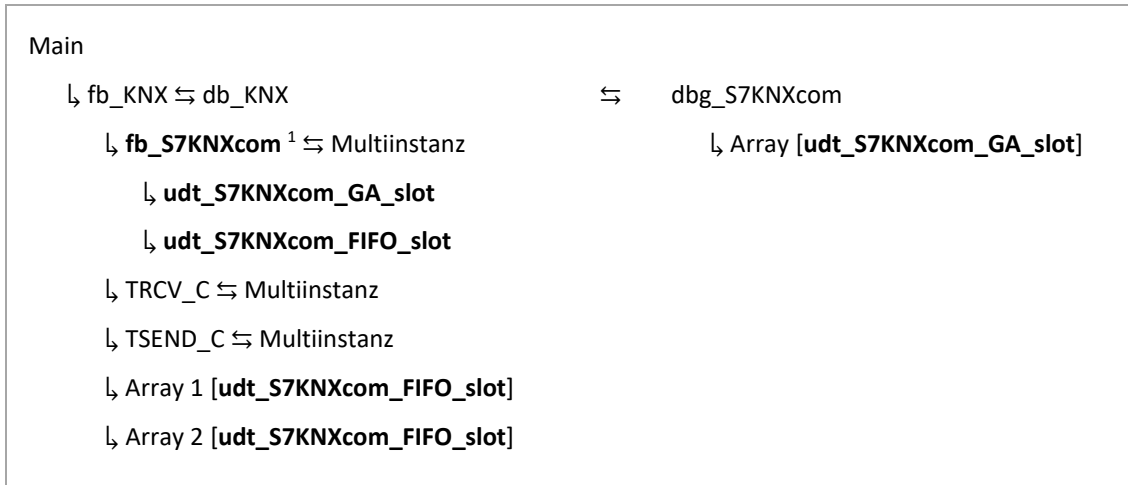
Abbildung 1 • S7KNXcom Programmstruktur
